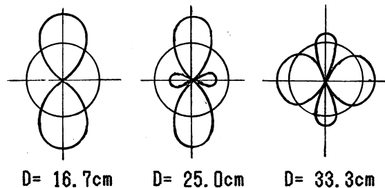
Dの距離による水平面電界指向性の変化図
