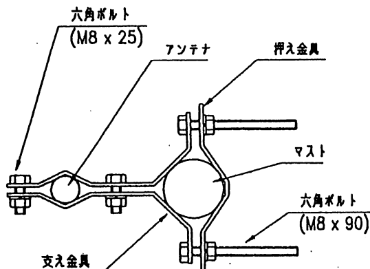
マストが40φより太い場合
