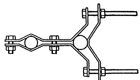
マストが40φより細い場合
