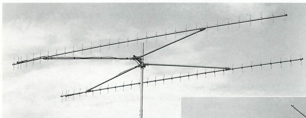
MACH-7 CYA-731W 430MHz31エレスタック
