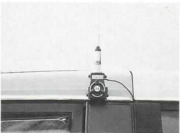
RS-80 ¥3,800 ●ヘビーデューティルーフ基台 ●ダイヤルロック10度ステップ18段階折曲機構付 ●シルバータイプもあり
