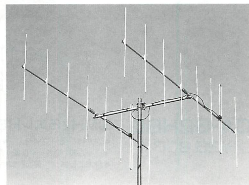
CYA-S208E 144MHz8エレスタック
