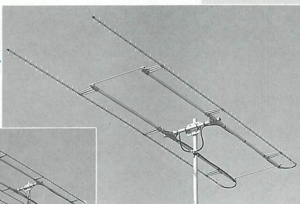
MACH-G1 CYA-1251W 1200MHz 51エレスタック
