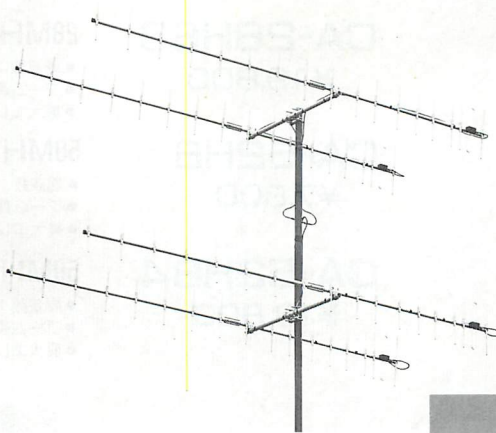
CYA-2S718E 430MHz18エレスタック2段
