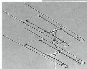
CYA-1251W2 1200MHz51エレスタック2段
