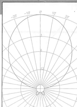
水平面指向性
