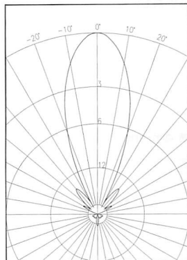
垂直面
