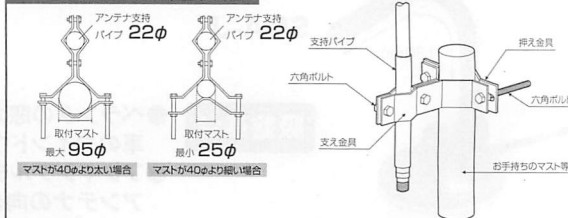
GHシリーズアンテナ取付金具(共通)
