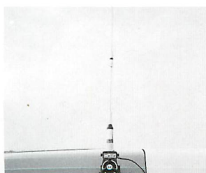
RS-20をルーフサイドに取り付ける
