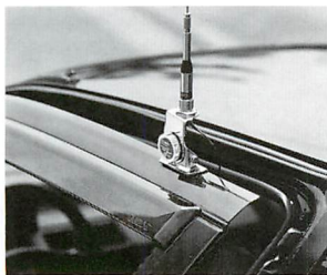
DORをドアフレームに取り付ける
