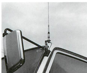
RS-4をミラーパイプに取り付ける
