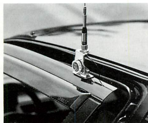
DORをドアフレームに取り付ける
