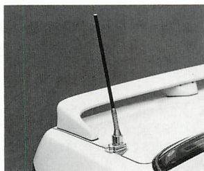
CRDをトランクに取り付ける
