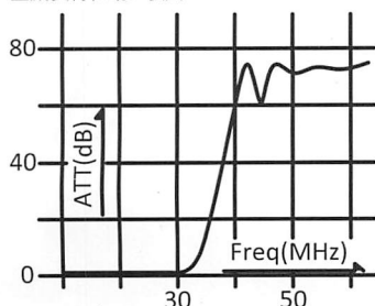
■減衰特性(参考値)
