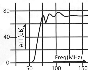
■減衰特性(参考値)
