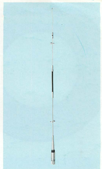
CX-807PM/N ¥7,500(折曲機構付) 144MHz \frac{1}{2} λCフェイズ 430MHz5/8λ2段 Cフェイズ 900MHz5/8λ4段Cフェイズ ●周波数：144/430/900MHz帯 (受信)800MHz帯対応 ●利得：3.15/6.3/8.7dB ●耐入力：120W 50W(900MHz) ●全長：1.0m ●重量：315g
